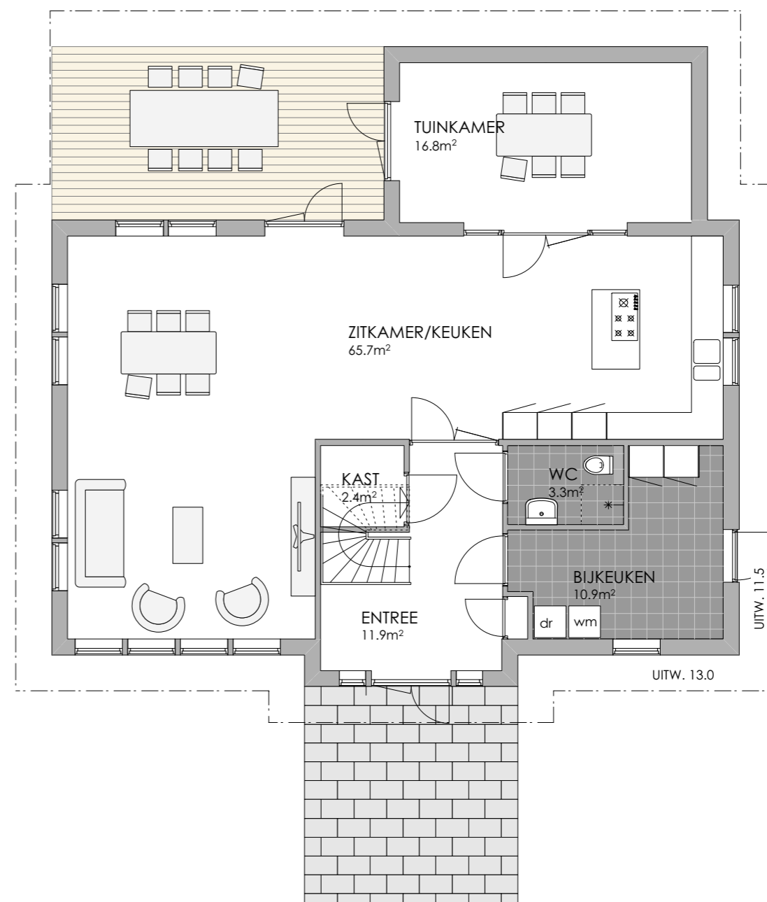
Begane grond
